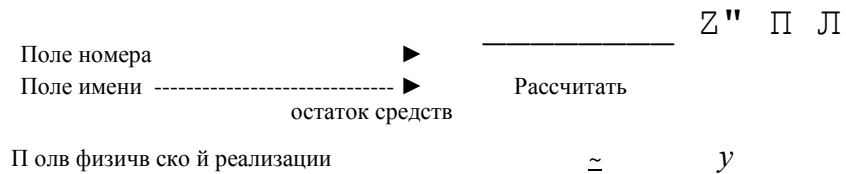
Рис. 5. Процесс
