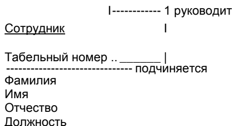
Рис. 13. Рекурсивная связь
